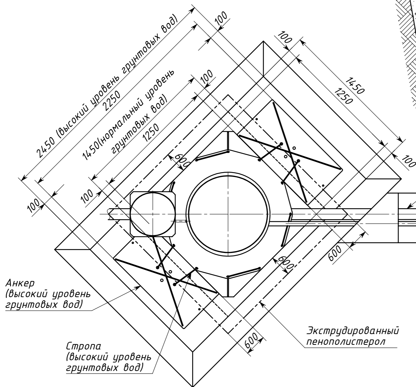
Вид сверху
